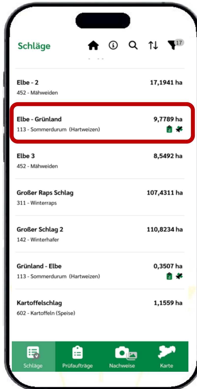
Abbildung 78: Schlagliste KALLE-App
