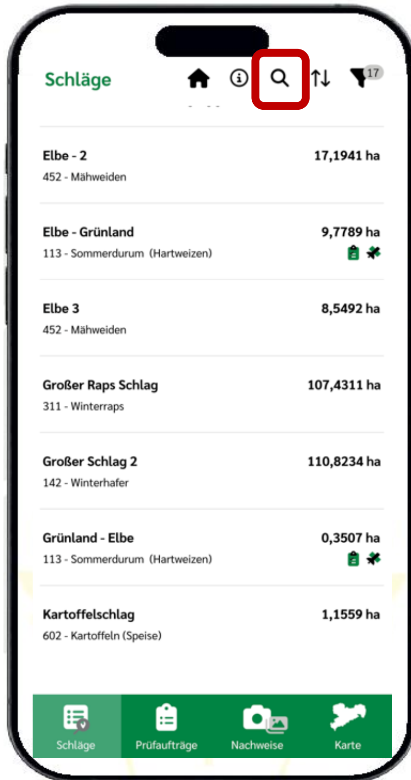
Abbildung 72: Schlagliste KALLE-App
