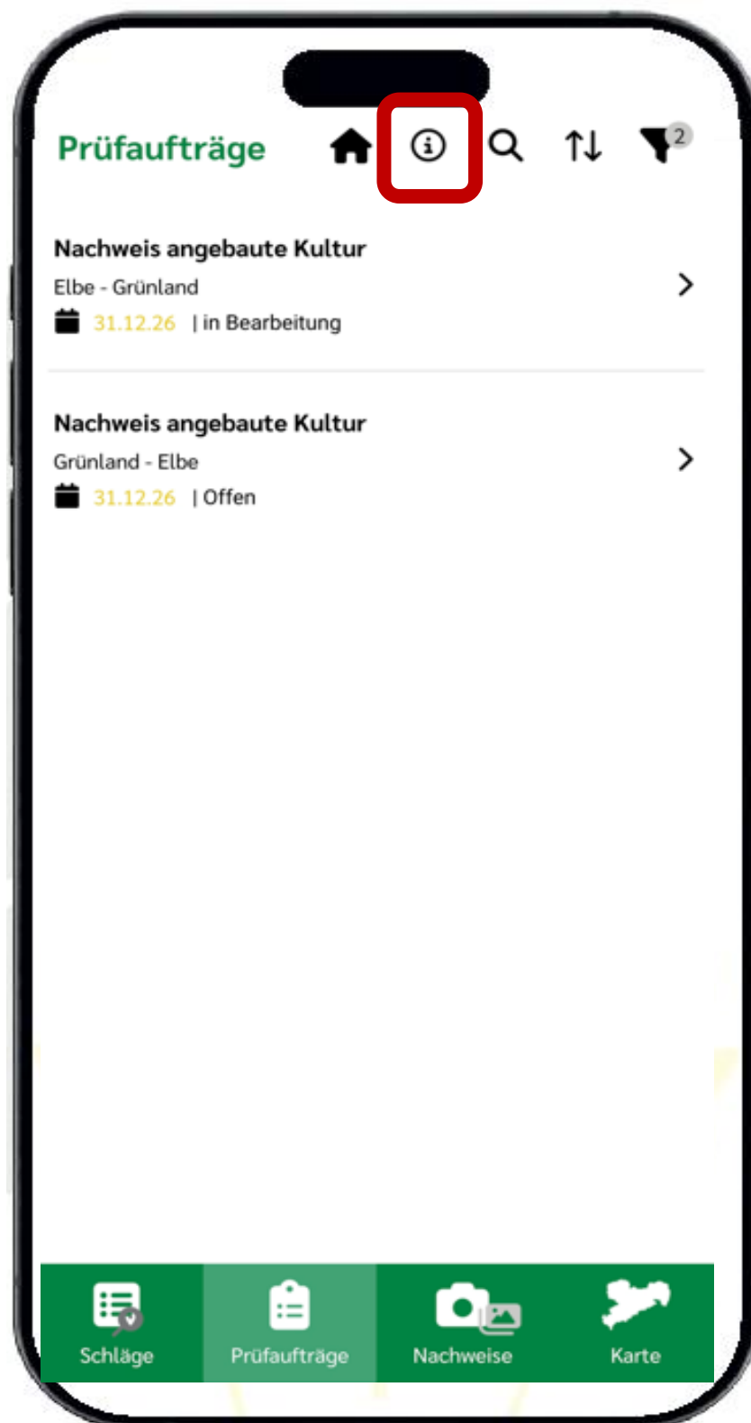
Abbildung 85: Prüfaufträge KALLE-App
