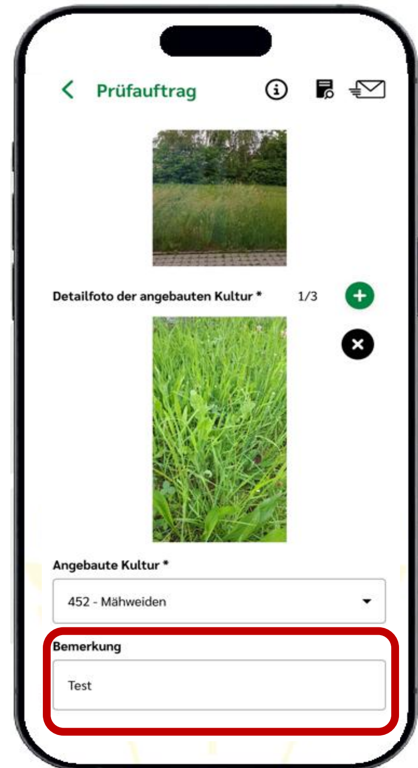
Abbildung 66: Prüfauftrag KALLE-App
