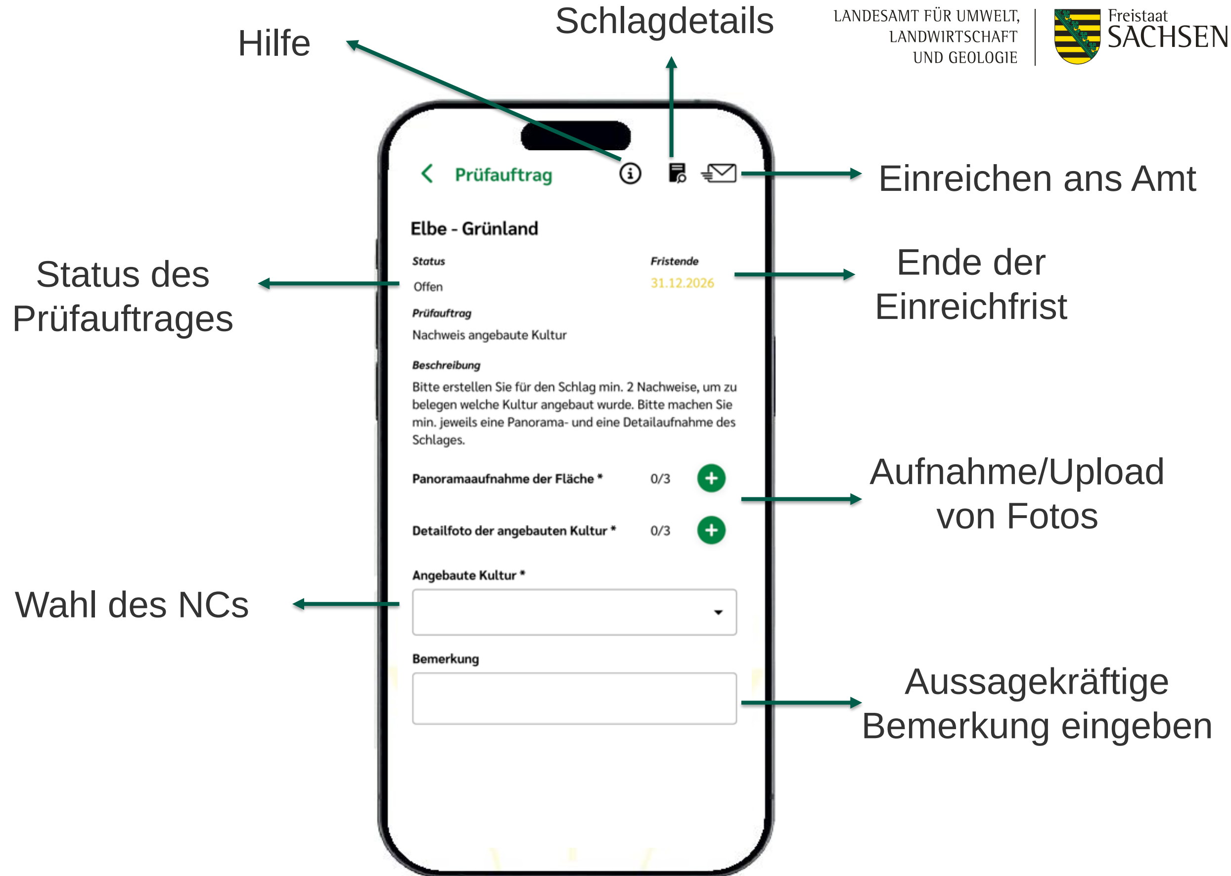
Abbildung 41: Prüfauftrag KALLE-App
