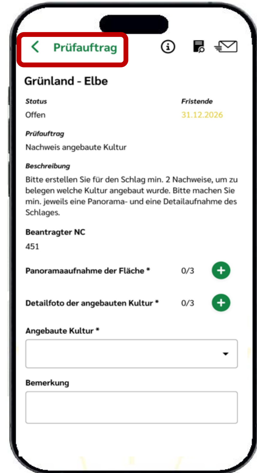
Abbildung 94: Prüfauftrag KALLE-App
