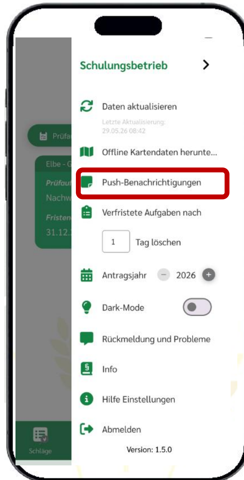
Abbildung 28: Einstellungen KALLE-App
