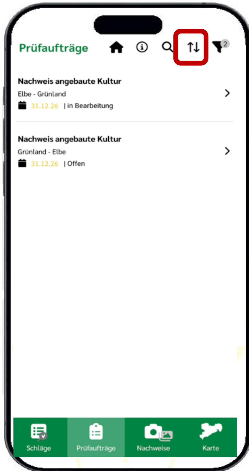
Abbildung 89: Prüfaufträge KALLE-App
