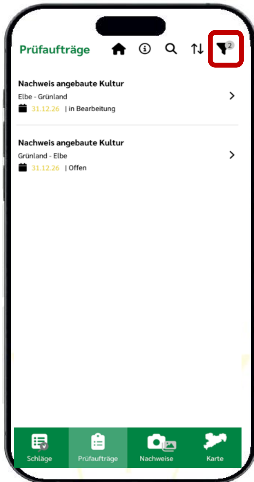
Abbildung 91: Prüfaufträge KALLE-App
