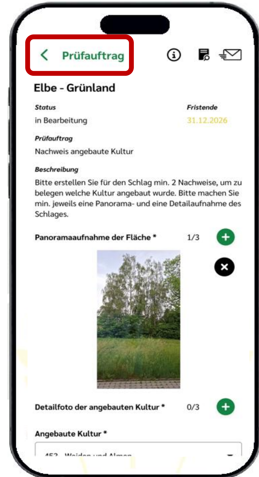
Abbildung 82: Prüfauftrag KALLE-App
