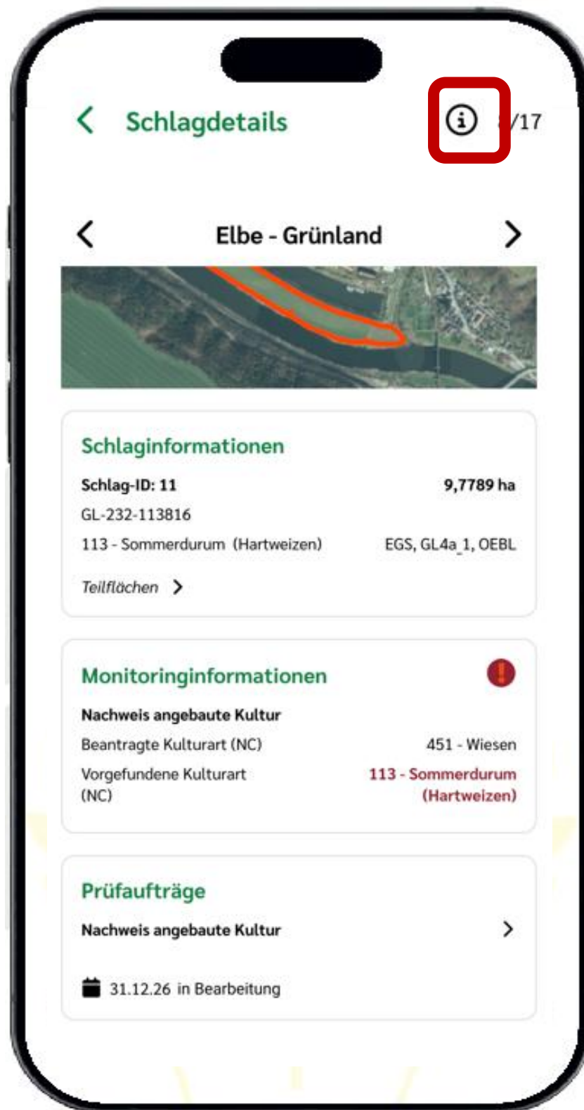
Abbildung 79: Schlagdetails KALLE-App
