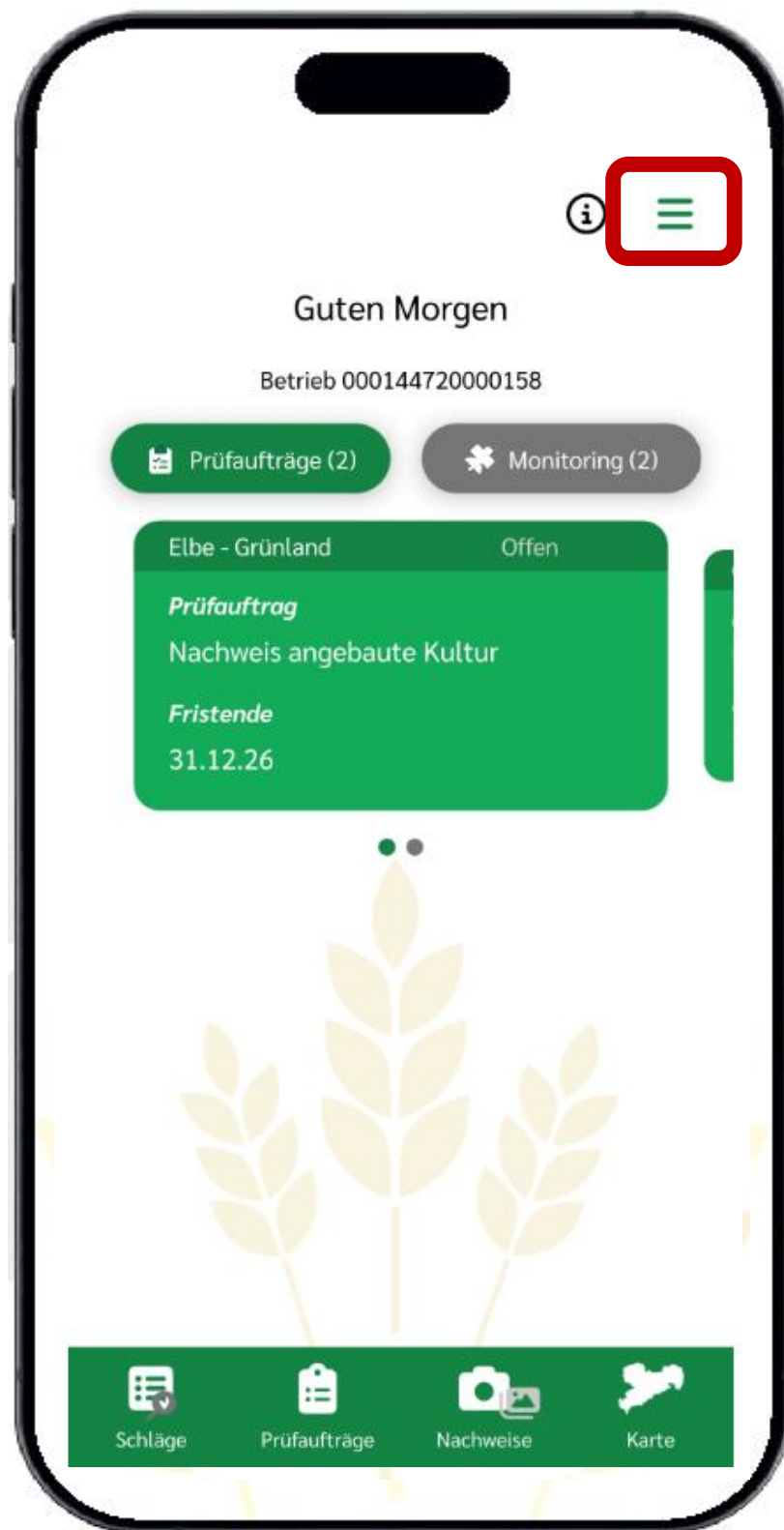
Abbildung 27: Dashboard KALLE-App
