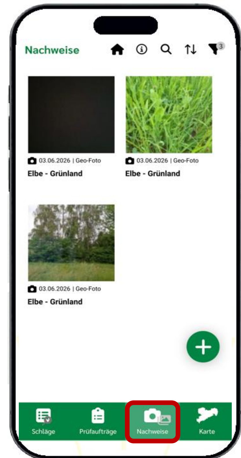
Abbildung 95: Nachweise KALLE-App
