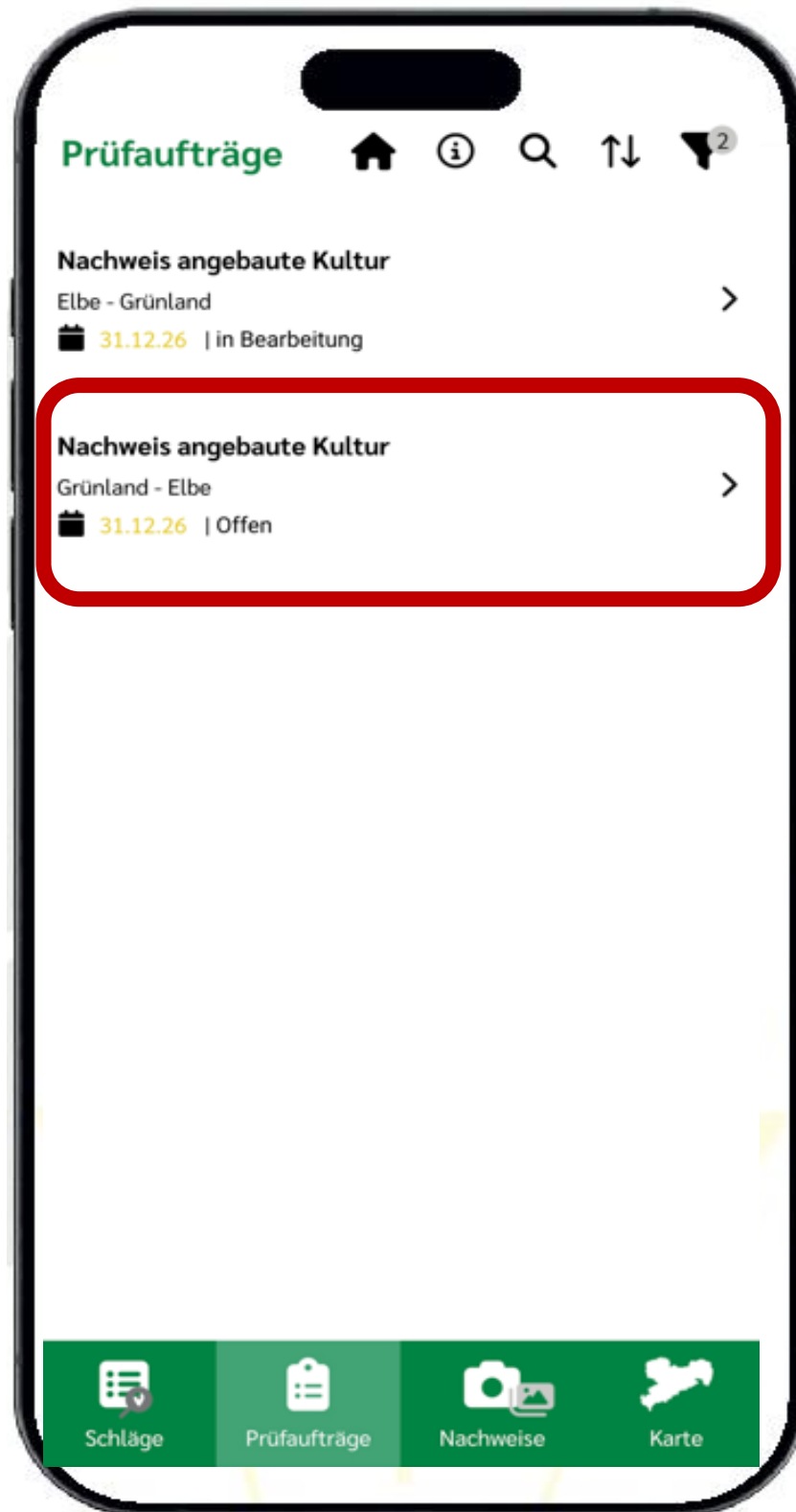
Abbildung 93: Prüfaufträge KALLE-App
